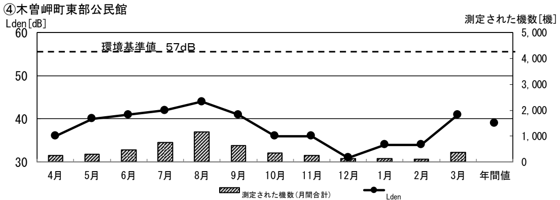
図 3-2 調査地点別の Lden 及び測定された機数
