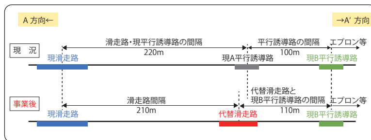
代替滑走路事業実施前後のA-A'方向の模式図(A-A'の方向は上の平面図参照)
